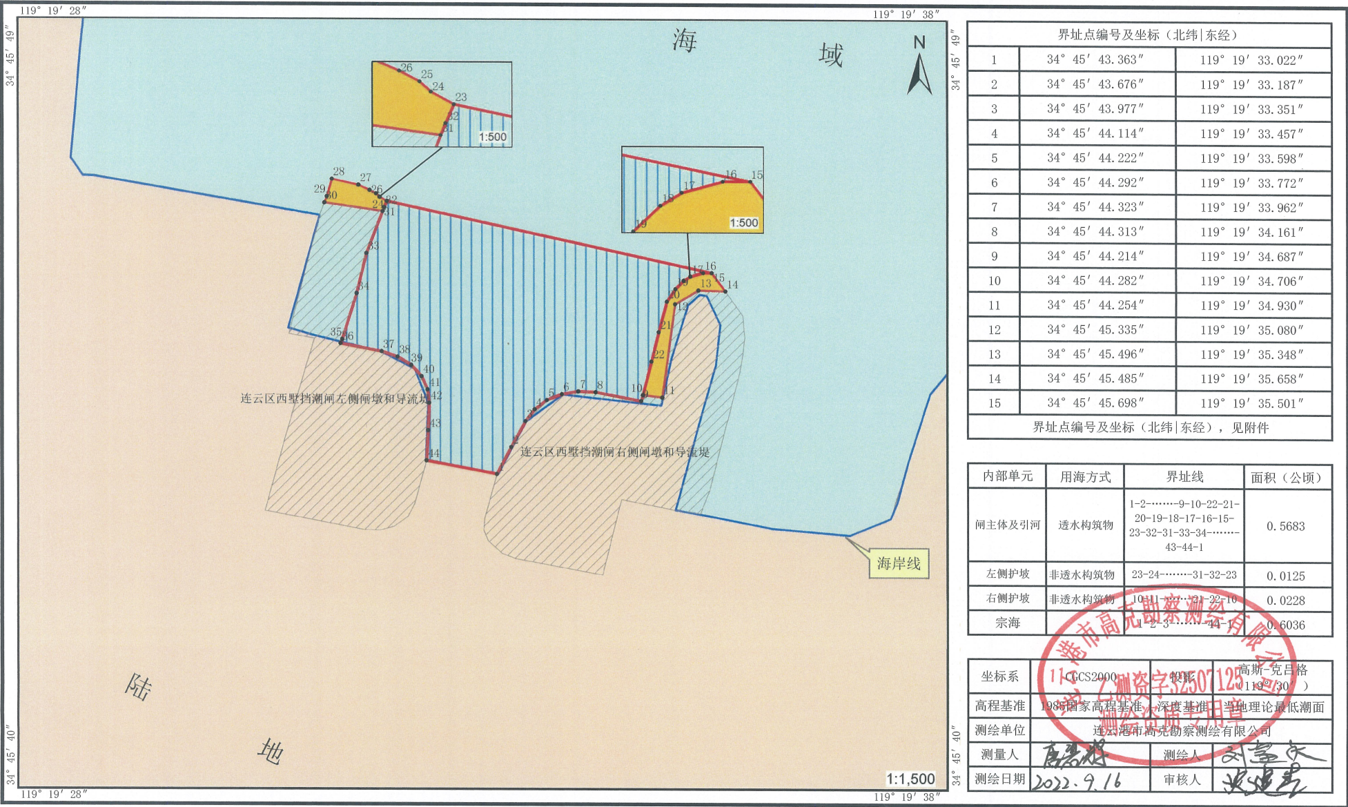
连云港市连云区西墅挡潮闸工程（闸主体及引河、护坡）宗海界址图
