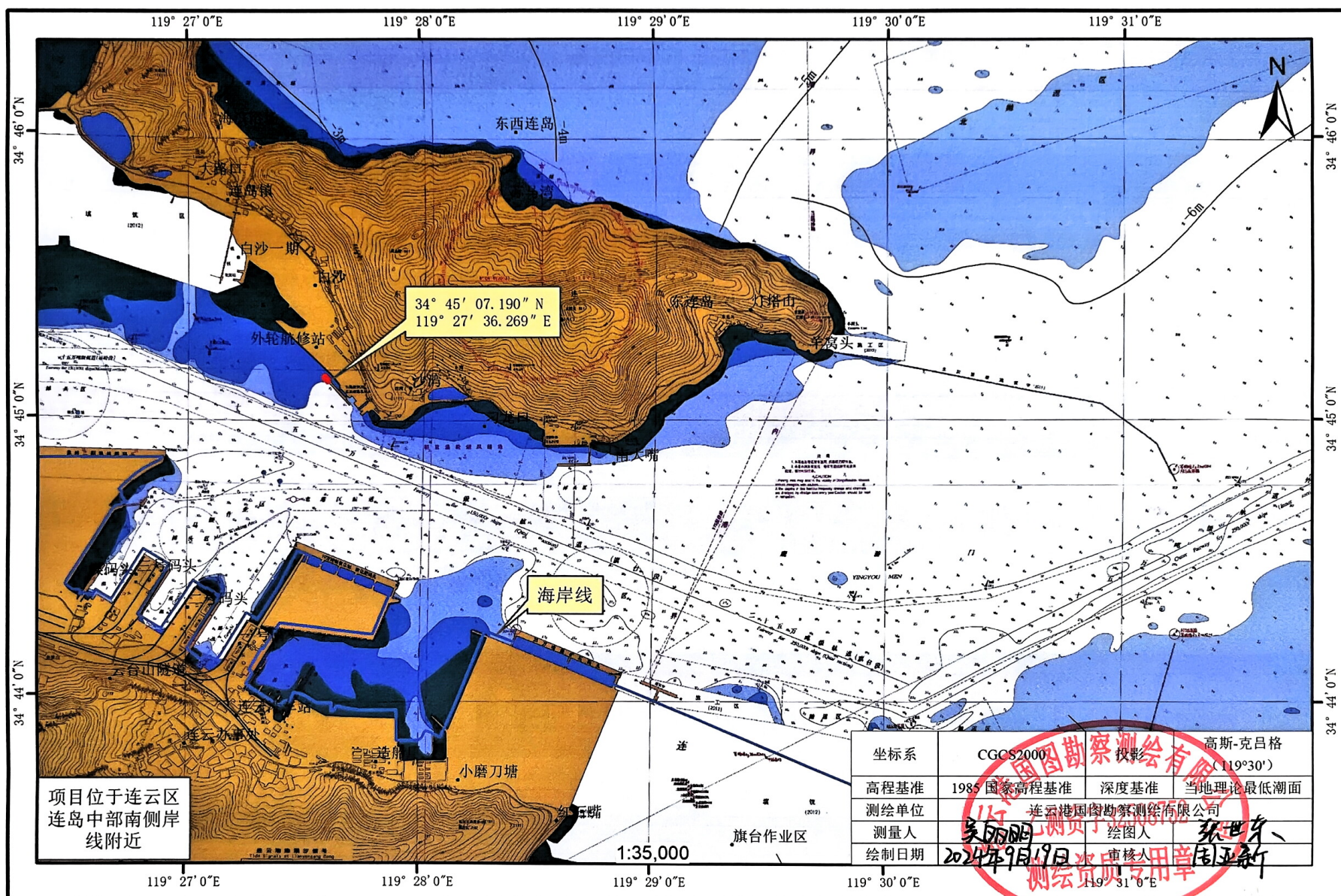
东海救助局连云港救助码头扩建工程宗海位置图
