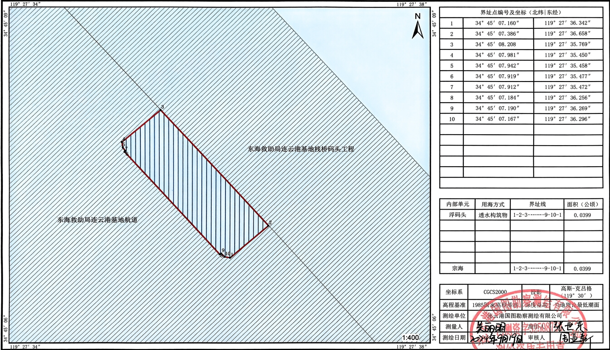
东海救助局连云港救助码头扩建工程宗海界址图
